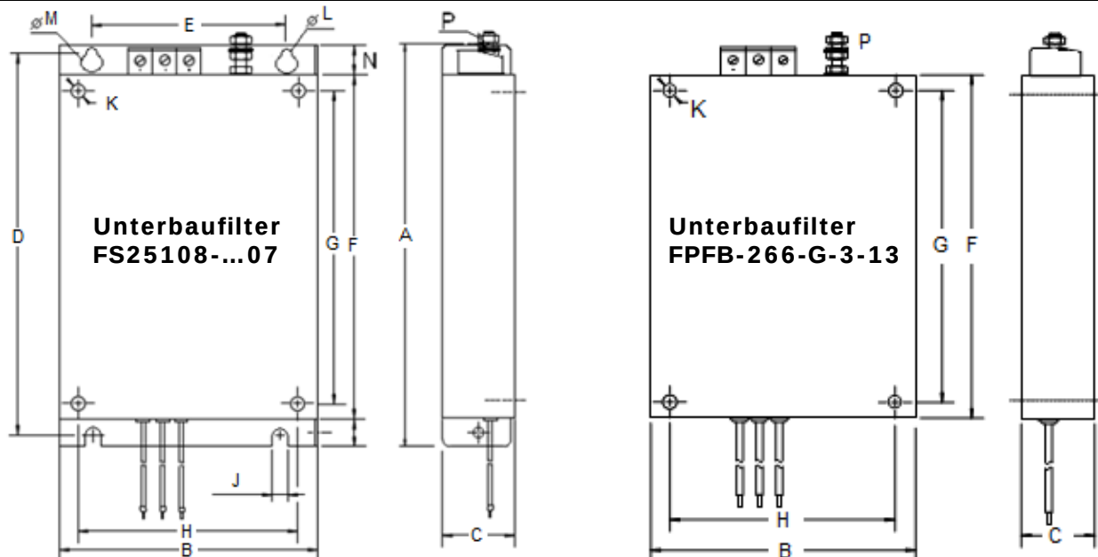
Abmessungen Nebenbaufilter [mm]
