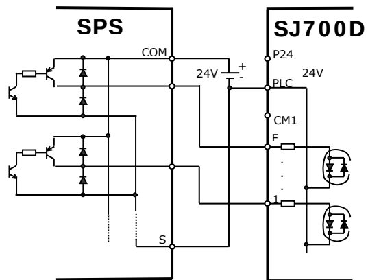
PNP-Logik Externe Steuerspannung
