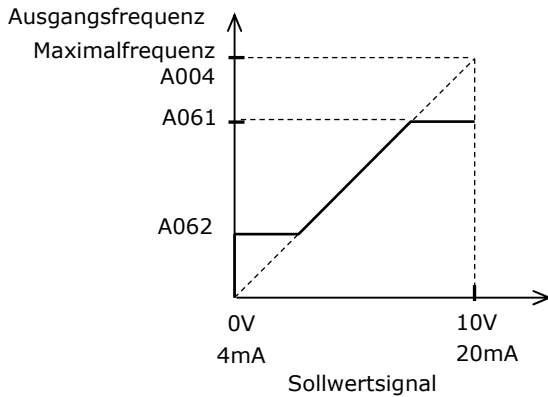
Sollwertvorgabe über Analog-Eingang O bzw. OI
