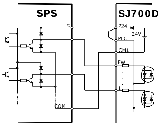
NPN-Logik Interne Steuerspannung
