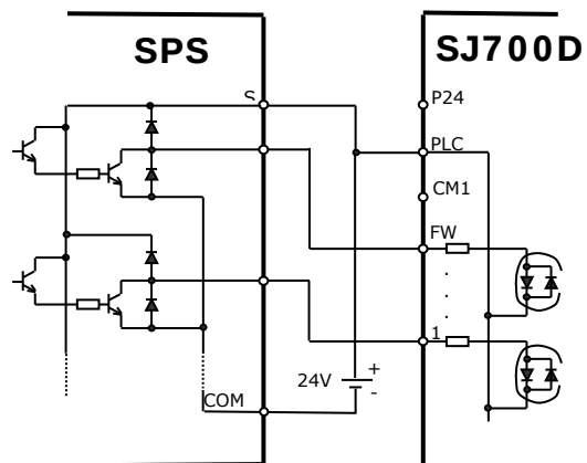
NPN-Logik Externe Steuerspannung
