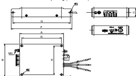
EMV-Filter - Dreiphasig (FPF-8123)
